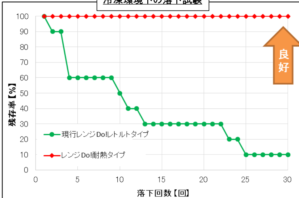
冷凍環境下の落下試験
