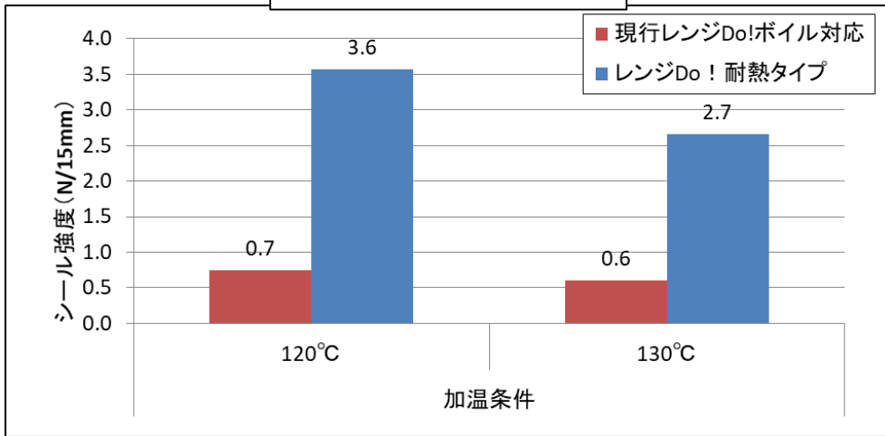
高温環境下のシール強度
